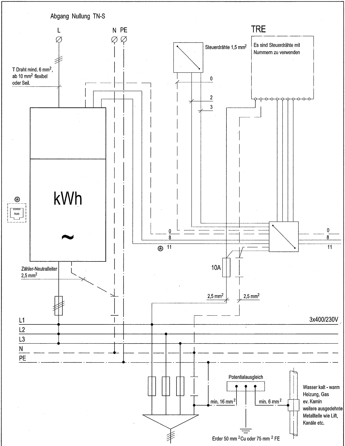
Schema Zähler Direktmessung ⊕ Nur bei Fernauslesung / Leistungsmessung
